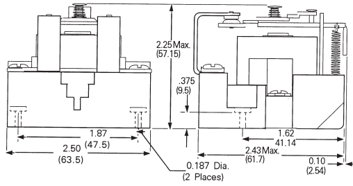
3TX7130 SPDT
