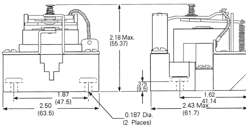
3TX7130 SPDT
